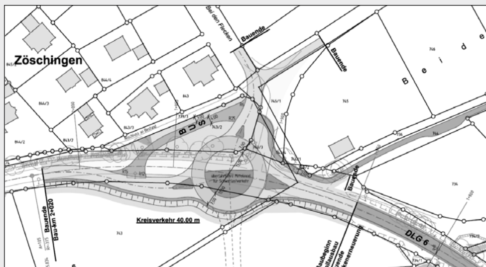
Detailskizze Kreisverkehr:
